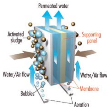
SCHEMA DI FUNZIONAMENTO DELLA FILTRAZIONE CON MODALITÀ DI FILTRAZIONE Conceptual drawing of filtration
