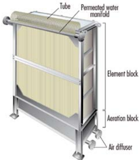
MODULO - Module
