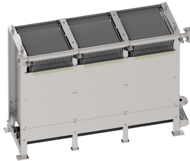
E-BOX MBR 03-105 Portata fino a 51 m 3 /d
