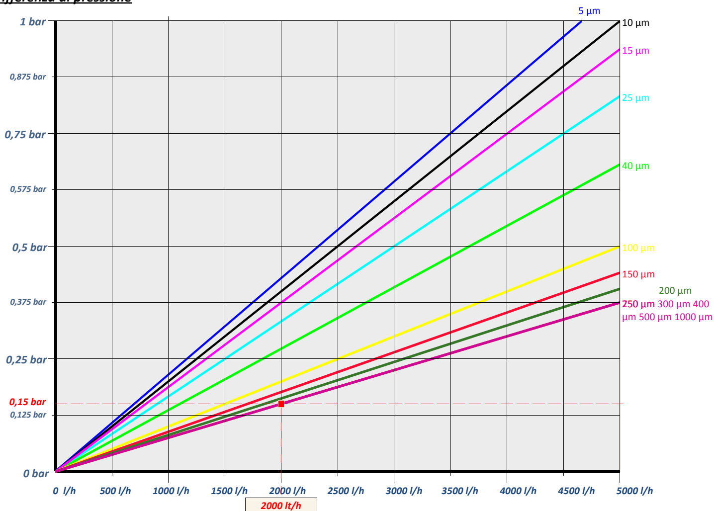
GRAFICO DELLE PORTATE (Litri/Ora) IN FUNZIONE DELLA DIFFERENZA DI PRESSIONE (Bar)
